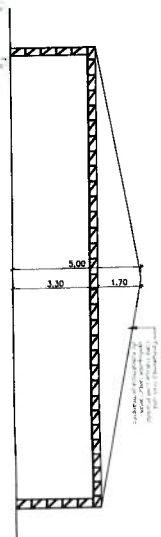
PALCO - CORTE B-B ESCALA 1:100
